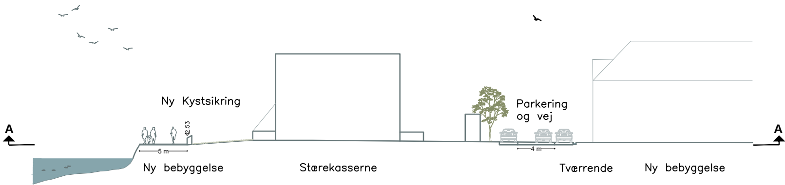
Principsnit gennem brygge, Stærekasserne og ny bebyggelse
