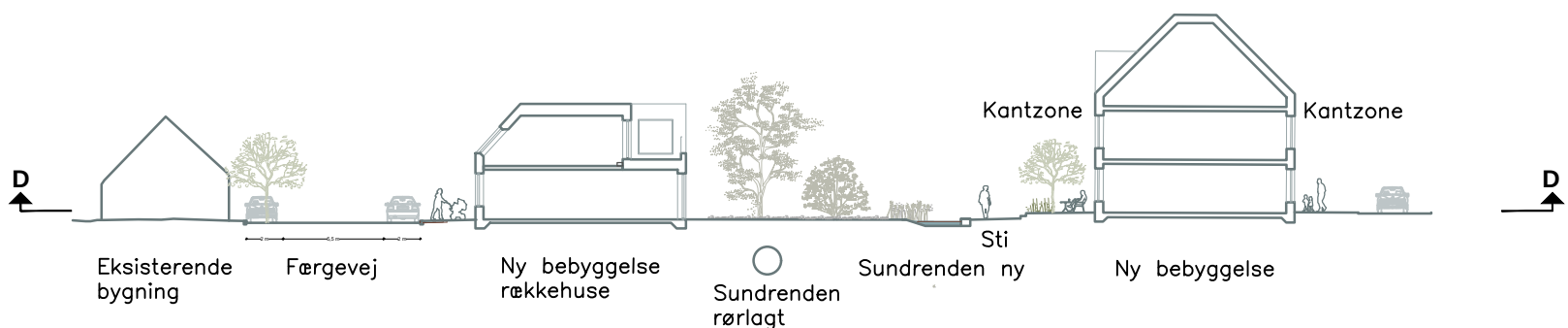
Principsnit gennem Sundrenden og rækkehuse
