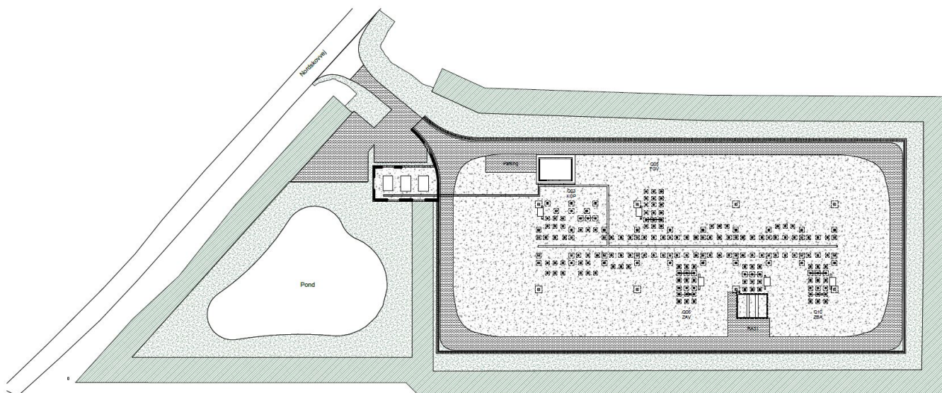
Situationsplan: Station Sdr. Højrup med det indhegnede stationsareal, regnvandsbassin og omkransende beplantningsbælte.
