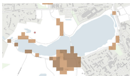
Lavbundskort (brun-orange)
