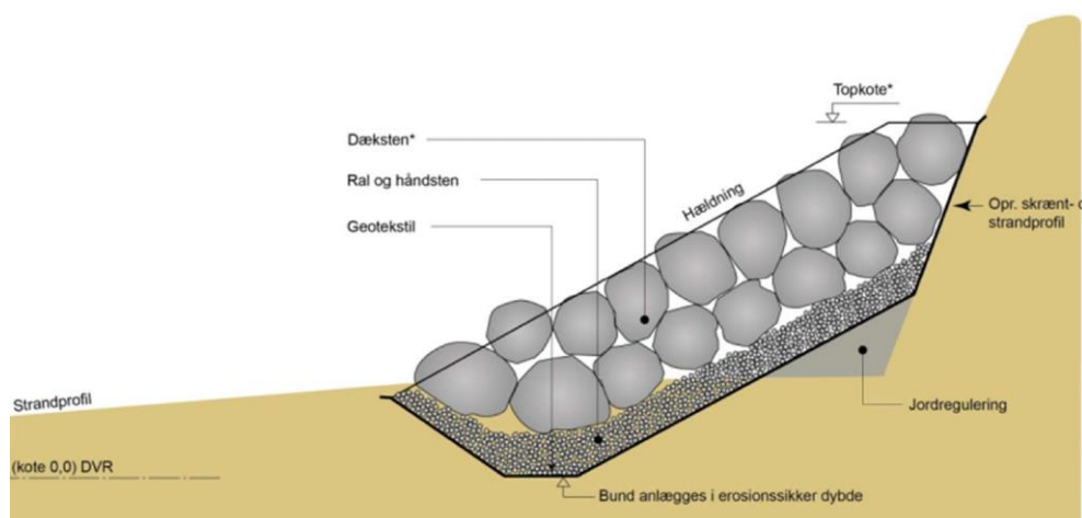
Figur 2, principtegning fra ansøgningen.
