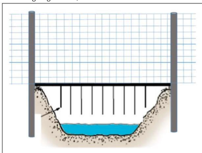
Figur 2: Principskitse for vandløbskrydsning med hængende stålør.
